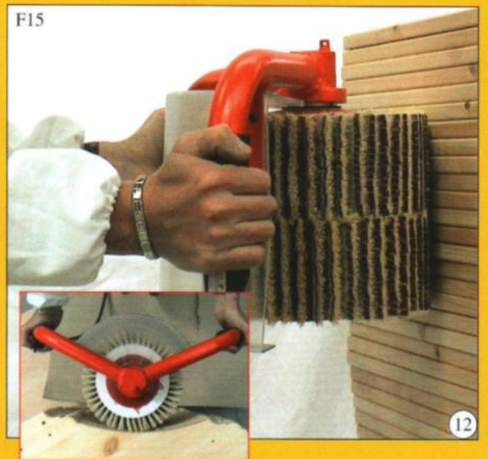
QT 300
